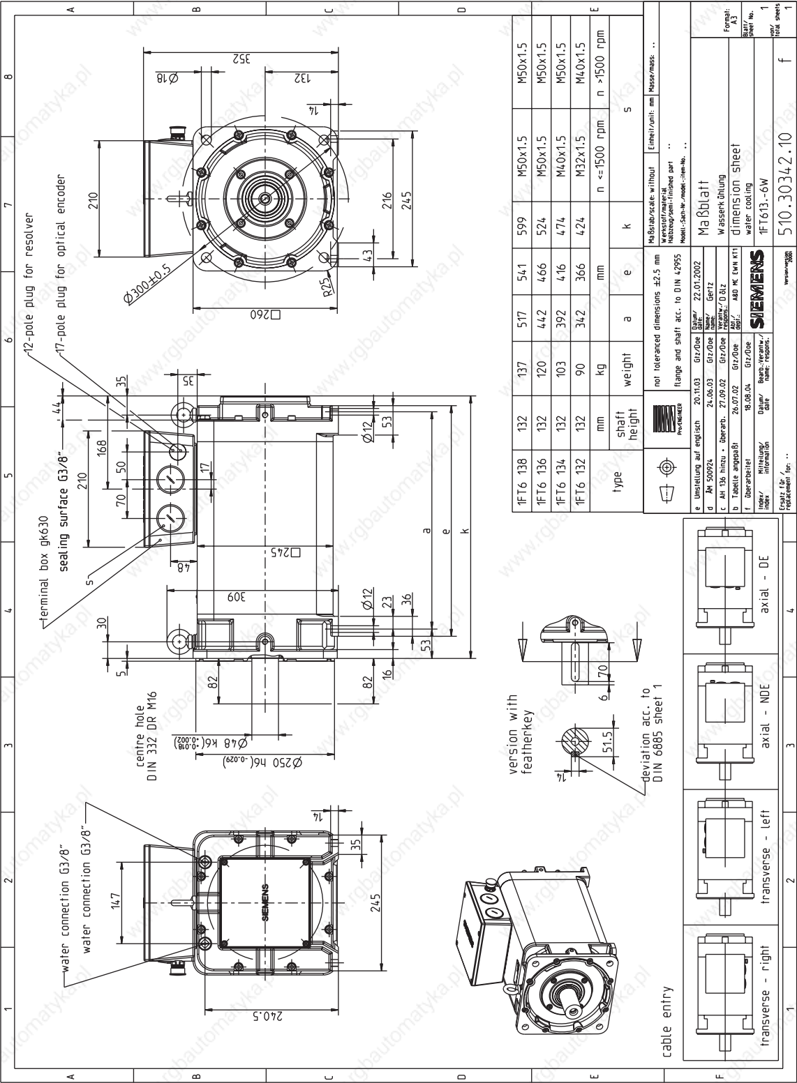
Figure 5-39 1FT613x-6Wx76-5xxx
