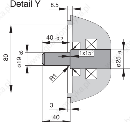
Detail Y
