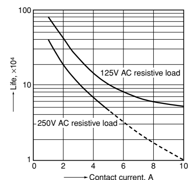
2. Life curve (N.O. side)
