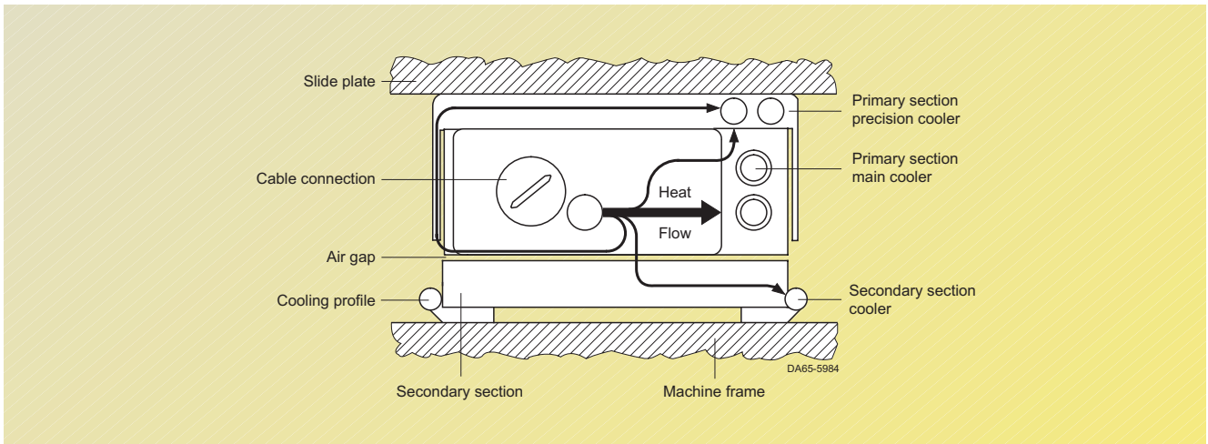
Fig. 4/11 Optional coolers
