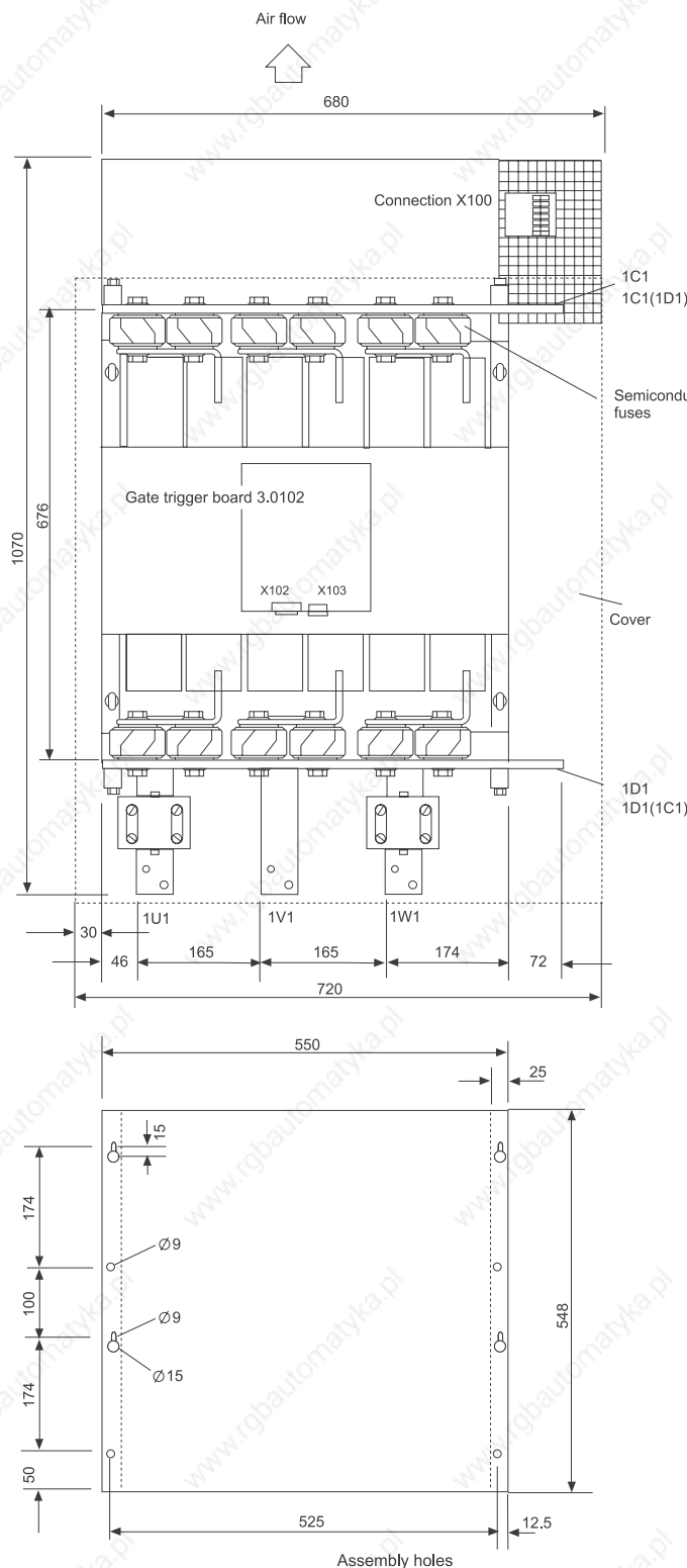
Abbildung 7: Dimensions power unit, size IV
