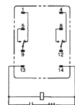
MY2-CR
