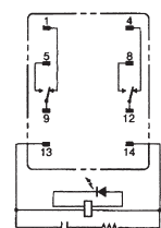
MY2N-CR
