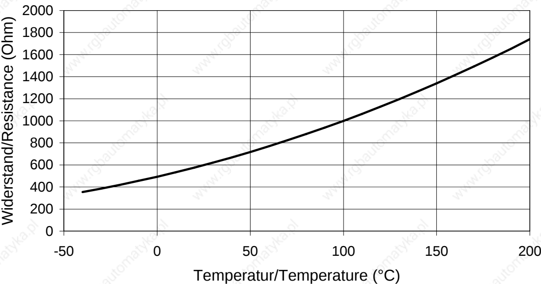
KTY84 - 130
