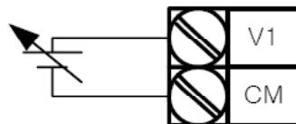
Zewnętrzne źródło sygnału 0~10
