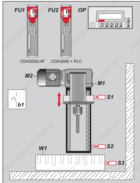
Bild: Bohrervorschubeinheit
