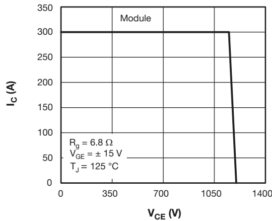
Fig. 5 - RBSOA
