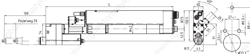
versetzter Abtrieb mit Motor-Umlenkgetriebe, 2 Messwertaufnehmer / Offset drive with reversible gears, twin transducer (redundant)
