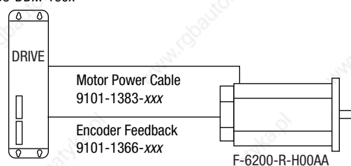
1398-DDM-150 1398-DDM-150x
