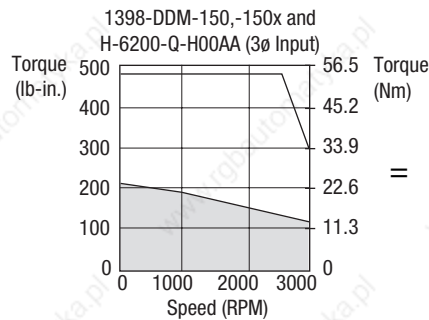
1398-DDM-150 1398-DDM-150x
