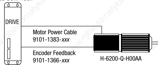
1398-DDM-150 1398-DDM-150x
