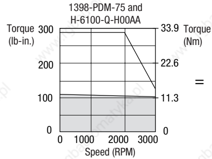
1398-PDM-75
