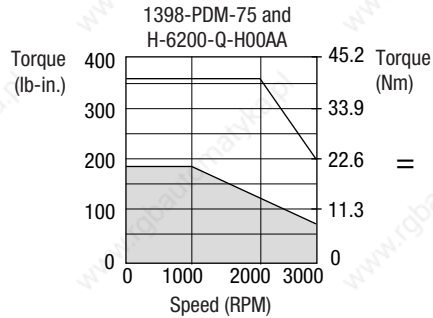
1398-PDM-75
