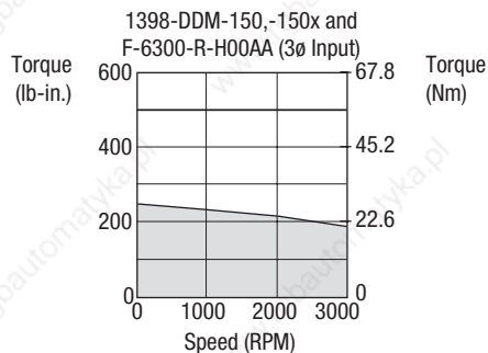
1398-DDM-150 1398-DDM-150x
