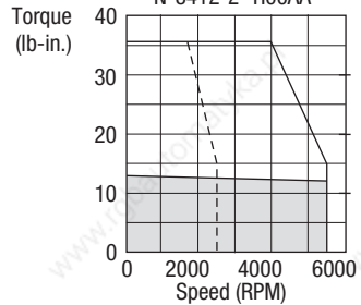
1398-DDM-009,-009x and N-3412-2-H00AA
