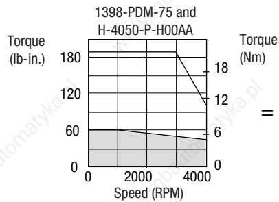
1398-PDM-75
