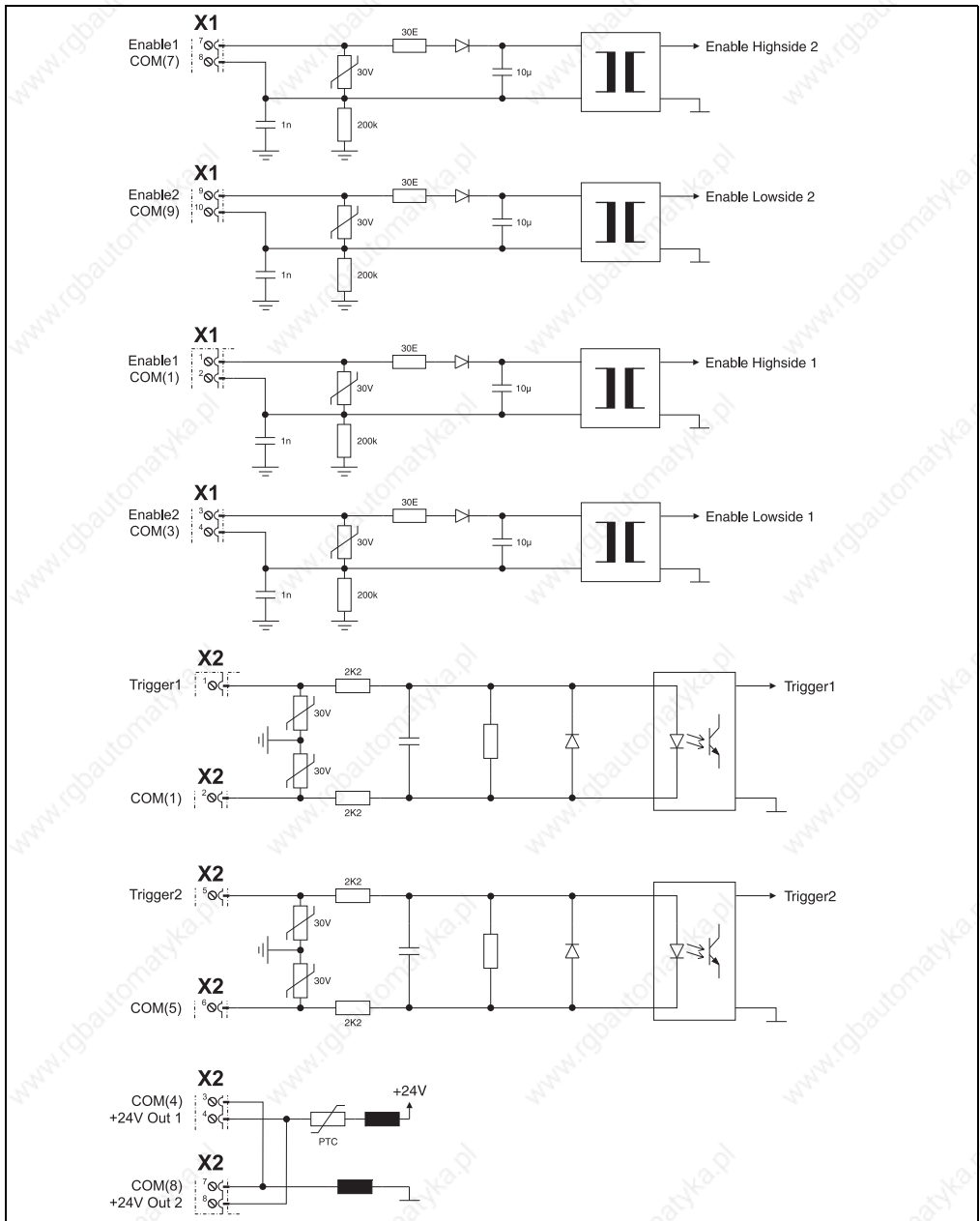
Figure 150: Input/output circuit diagram - 8BVI0014HxD0.000-1, 8BVI0028HxD0.000-1, 8BVI0055HxD0.000-1
