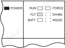
Dioda DH485 na procesorze SLC 5/03 jest obecnie oznakowana „DH+” na SLC 5/04
