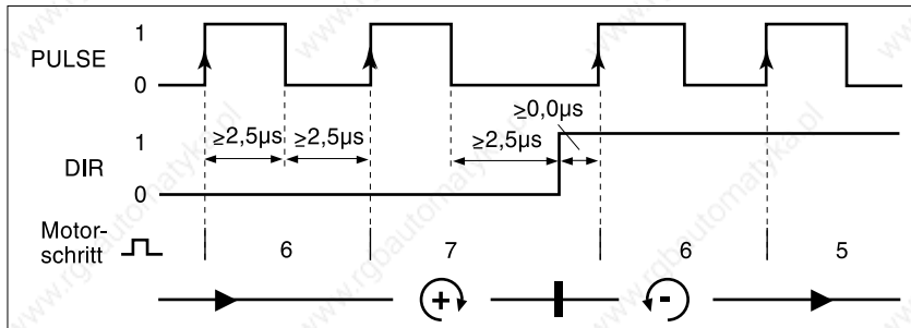
Bild 4.23 Pulse-Richtungs-Signal
