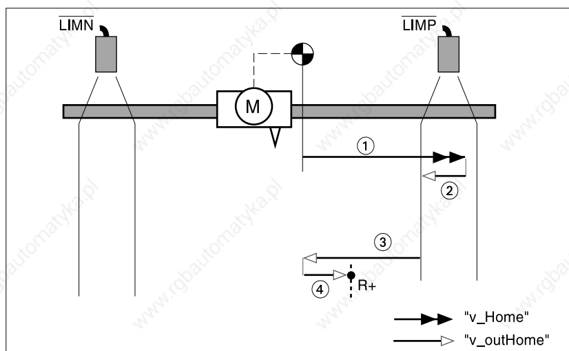
Bild 6.16 Referenzfahrt auf Endschalter
