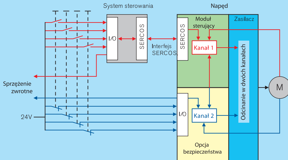
Wybór i sygnał sprzężenia zwrotnego za pośrednictwem komunikacji modułów sterujących (kanał 1) oraz sygnałów 24 V (kanał 2) – dla uproszczenia okablowania
