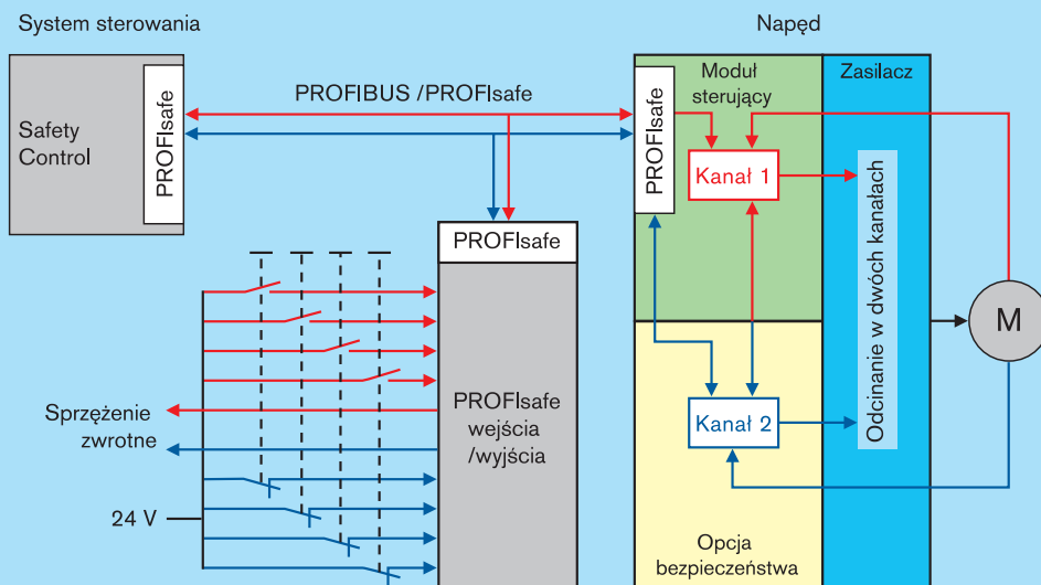
Wybór i sygnał sprzężenia zwrotnego za pośrednictwem interfejsu PROFIsafe – rozwiązanie przyjazne dla użytkownika
