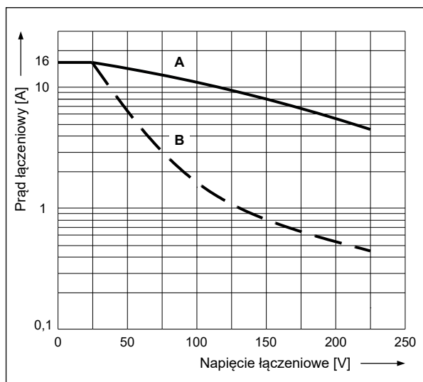
Maks. zdolność łączeniowa dla prądu stałego A - obciążenie rezystancyjne DC1 B - obciążenie indukcyjne L/R = 40 ms Un = 24 V DC - wersja 2Z (3 mm) Wykres 4
