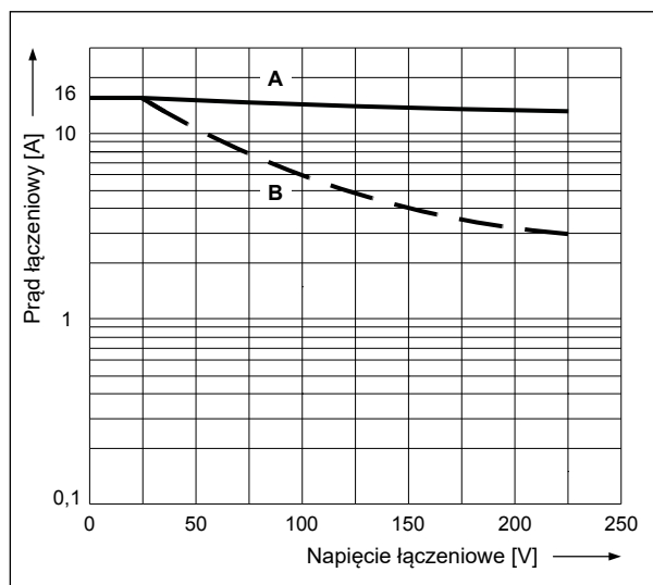
Maks. zdolność łączeniowa dla prądu stałego A - obciążenie rezystancyjne DC1 B - obciążenie indukcyjne L/R = 40 ms Un = 24 V DC - wersja 1Z (6 mm) Wykres 3
