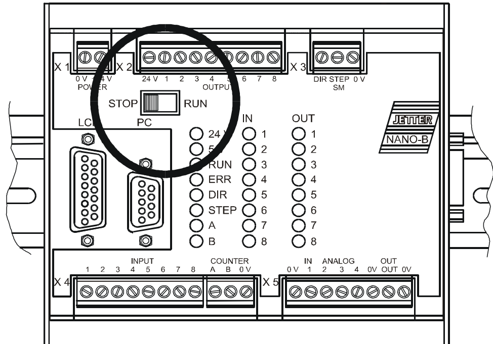
Fig. 16: STOP/RUN Switch
