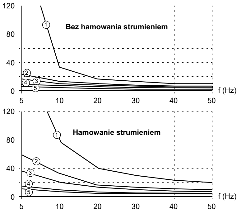
Rysunek 6-15 Moment hamujący silnika w procentach znamionowego momentu obrotowego w funkcji częstotliwości wyjściowej
