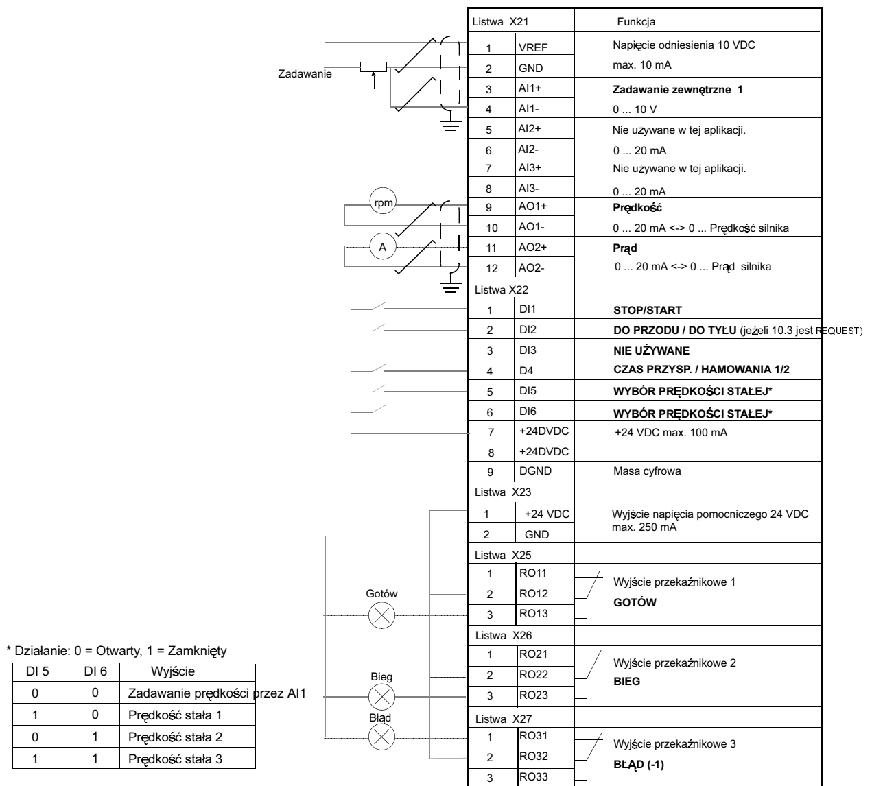
Rysunek 5-2 : Połączenia sterujące dla Makroaplikacji 1 - FABRYKA. Oznaczenia złącz płyty NIOC przedstawiono powyżej. W ACS 601 i ACS 604 połączenia użytkownika są zawsze wykonane bezpośrednio do zacisków wejścia i wyjścia płyty NIOC . W ACS 607 połączenia te są wykonywane albo bezpośrednio do płyty NIOC albo zaciski We/Wy płyty NIOC są wyprowadzone na oddzielną listwę przeznaczoną na połączenia użytkownika - właściwe oznaczenia zacisków patrz odpowiedni podręcznik instalacji i uruchamiania.
