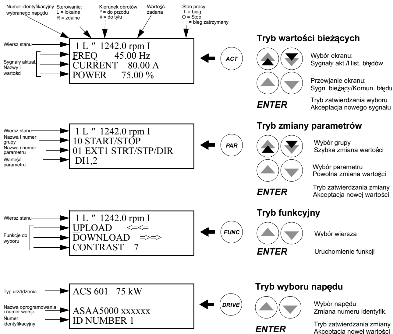
Rysunek 2-2 : Komunikaty na wyświetlaczu oraz funkcje klawiszy Panelu Sterowania.
