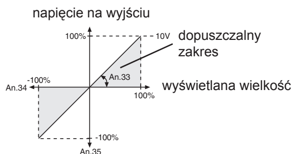
Rys. 6.2.14.a Ustawienie domyślne: brak przesunięcia, nachylenie 1
