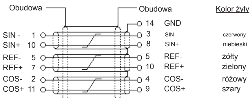
Rys. 6.10.2.c Kabel podłaczeniowy resolwera
