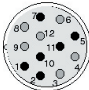
Rys. 6.10.2.c Kabel podłaczeniowy resolwera
