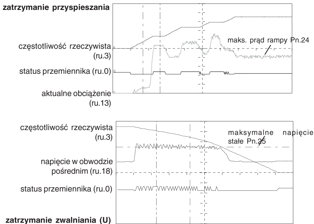
Ryc. 6.7.1.b Przykłady funkcji zatrzymania na rampie
