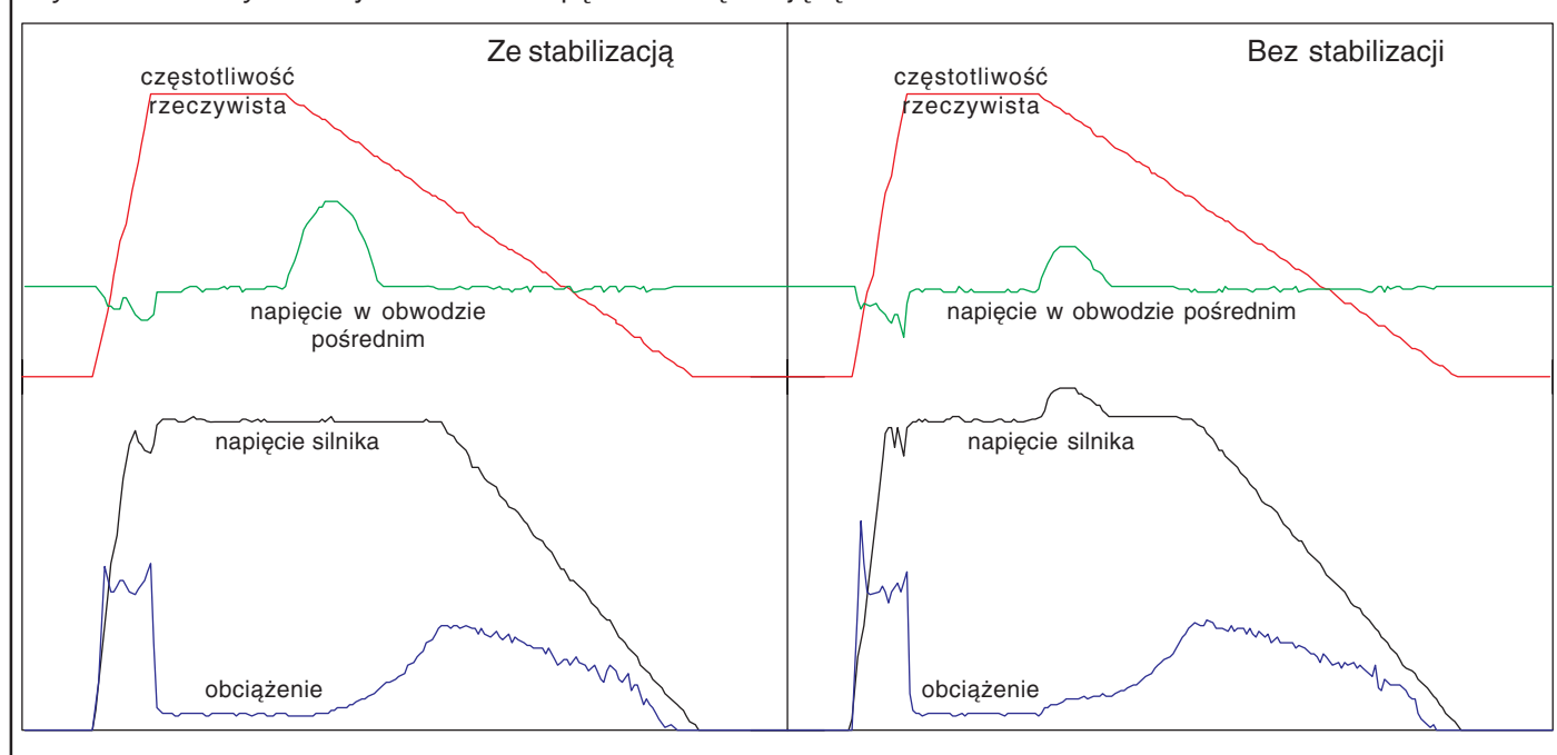
Ryc. 6.5.5.c Przykład: Wyhamowanie napędu z masą wirującą z 80Hz
