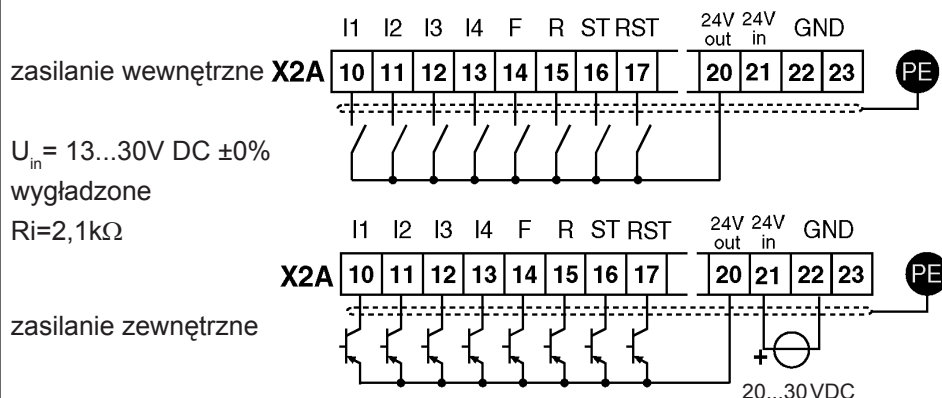
Ryc. 6.3.2.a Cyfrowe wejścia w układzie sterowania PNP (di.0 = 0)
