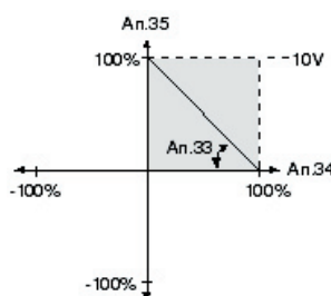
Rys. 6.2.14.b Odwrócenie wyjścia analogowego
