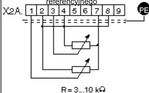
Rys. 6.2.2.b Sterowanie za pomocą potencjometru oraz wewnętrznego napięcia referencyjnego
