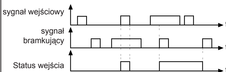
Ryc. 6.3.8.c Strob statyczny, tryb 2 (di.7 = 2)
