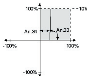
Rys. 6.2.14.c Wyjście analogowe jako przełącznik
