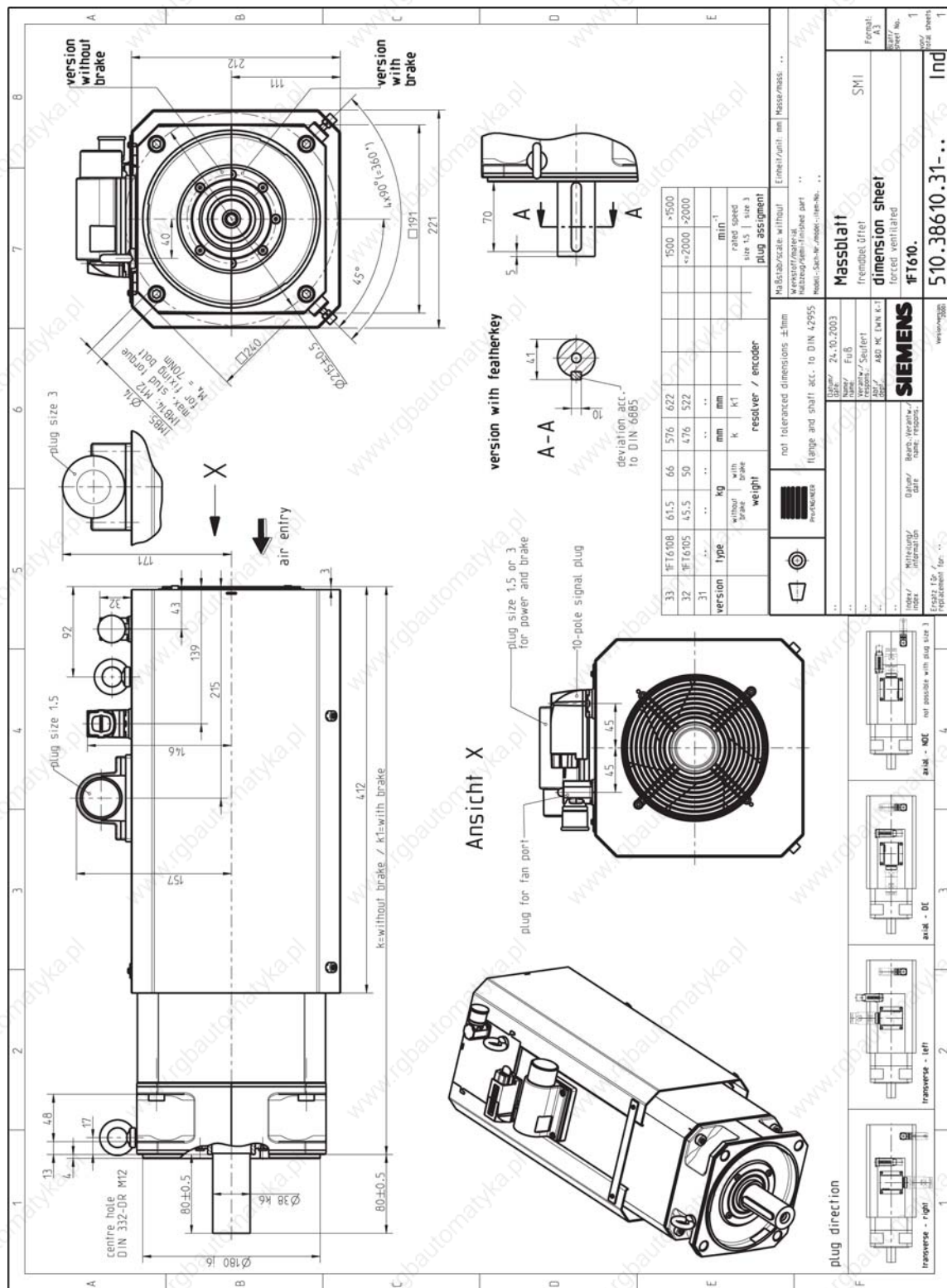
Figure 5-10 1FT610□-□S□plug□DQ
