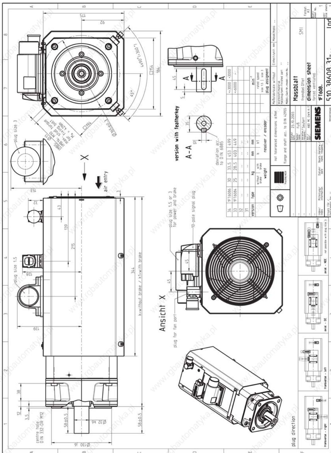
Figure 5-9 1FT608□-□S□DQ
