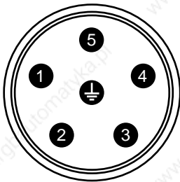
SOURIAU 8GN-QL2-6P
