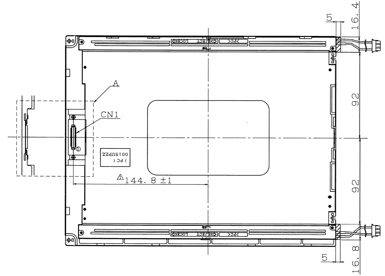
FIG1 LQ121S1DG11 OUTLINE DEMENSIONS
