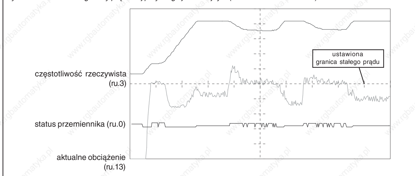
Ryc. 6.7.2 Działanie granicy prądowej przy biegu jednostajnym (ustawienie standardowe)
