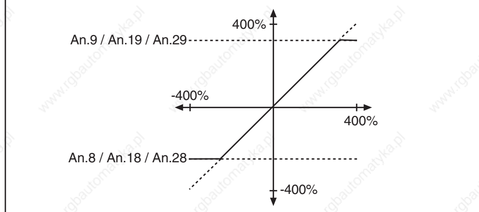
Rys. 6.2.8 Ograniczanie sygnału analogowego
