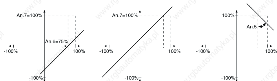
Rys. 6.2.7.c Offset X (An.6)=75%; Y-Offset (An.7)= 100%; Wzmacnienie (An.5)= -1.00
