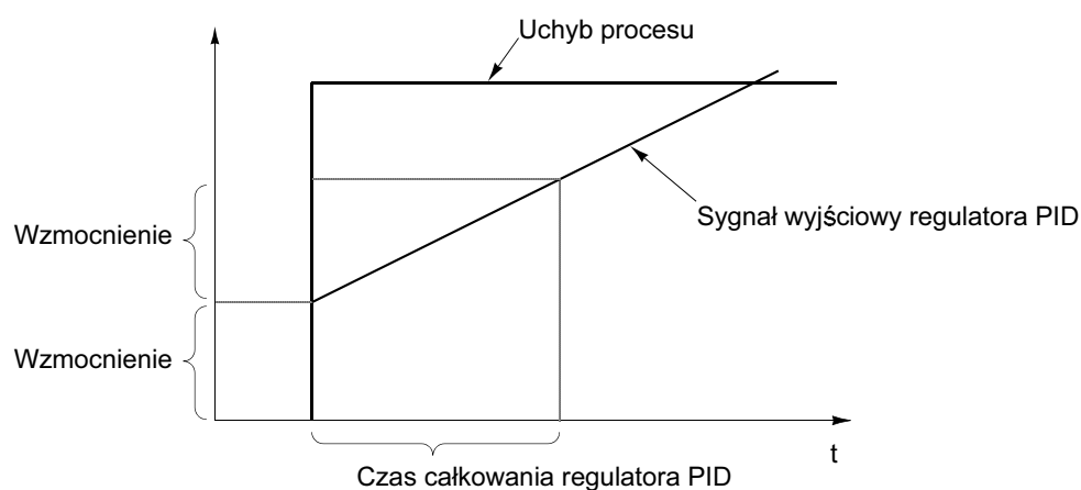
Rysunek 6-22 Wzmacnienie regulatora PID , czas całkowania i uchyb.
