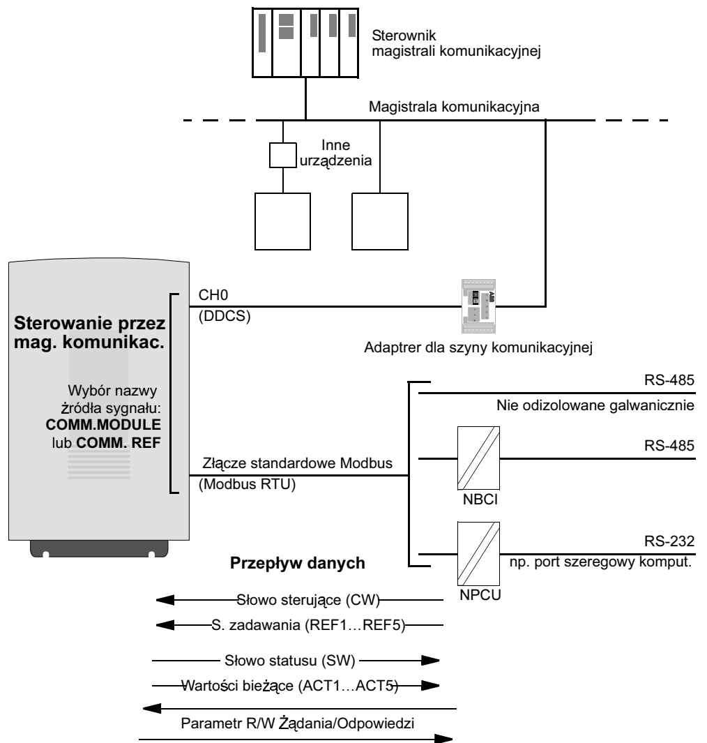
Rysunek C-1 Sterowanie przez magistralę komunikacyjną.
