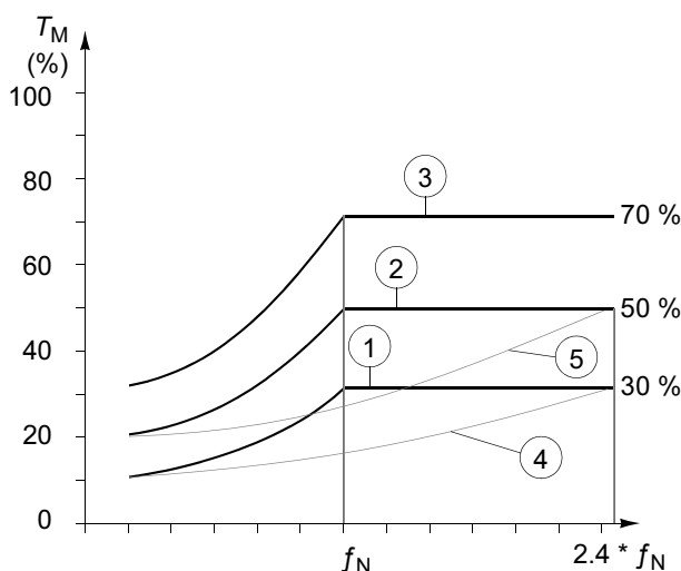
Rysunek 6-21 Typy krzywych niedociążenia. T_M = znamionowy moment obrotowy silnika; , f_N = znamionowa częstotliwość silnika.
