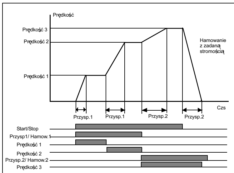
Przykład sterowania sekwencyjnego używającego stałych prędkości oraz różnych stromości przyspieszenia / hamowania
