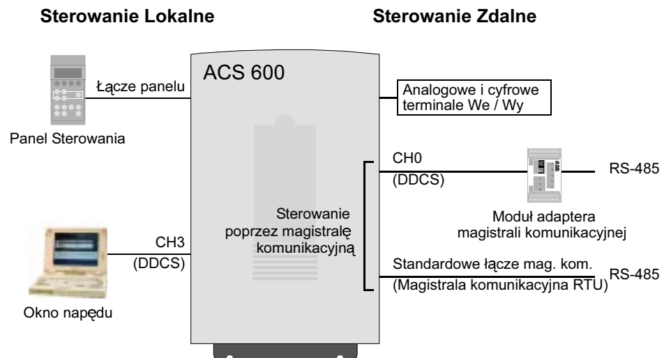
Rysunek 4-1 Sterowanie lokalne i zdalne.
