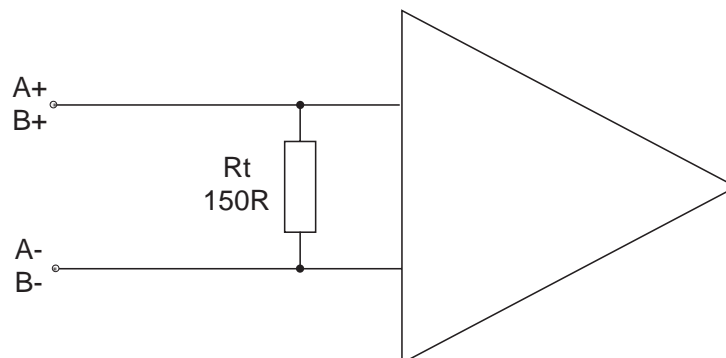
Fig. 6.10.2.b Input wiring of encoder inputs
