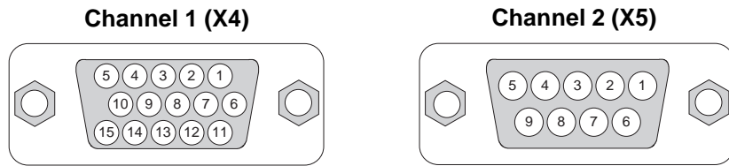
Fig. 6.10.2.a Incremental encoder inputs
