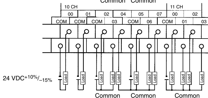
CPM1A-30CDT-□(-V1)
