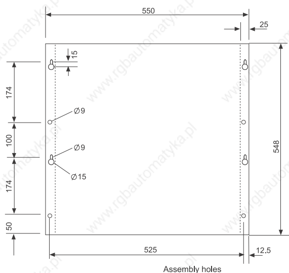
Abbildung 7: Dimensions power unit, size IV
