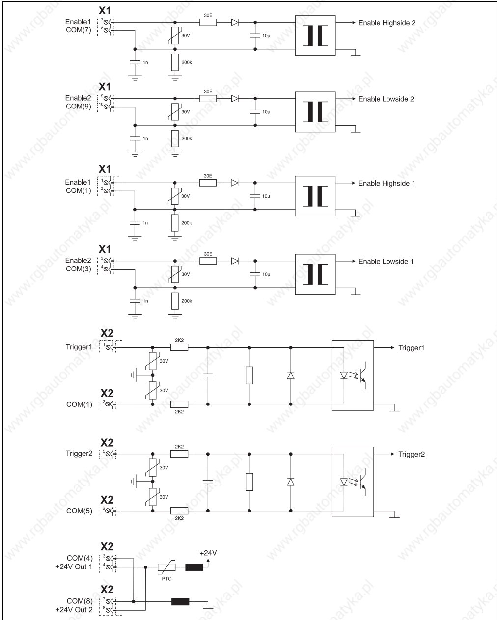
Figure 150: Input/output circuit diagram - 8BVI0014HxD0.000-1, 8BVI0028HxD0.000-1, 8BVI0055HxD0.000-
