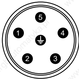
SOURIAU 8GN-QL2-6P
