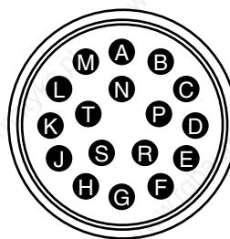
MS3102E-20-29P
