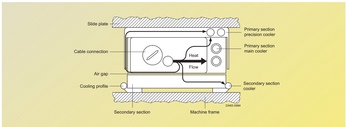
Fig. 4/11 Optional coolers
