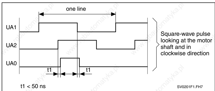
Fig. 4-127: Signal for incremental actual position value output
