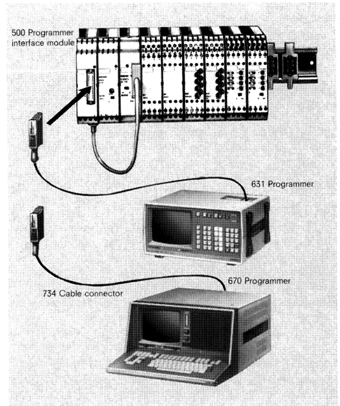
Fig. 11 500 Programmer interface module
