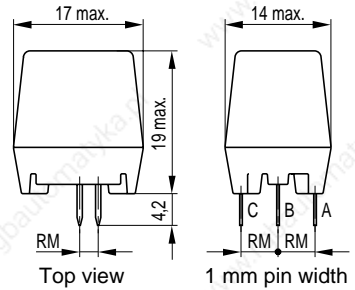
TPT0606-T
