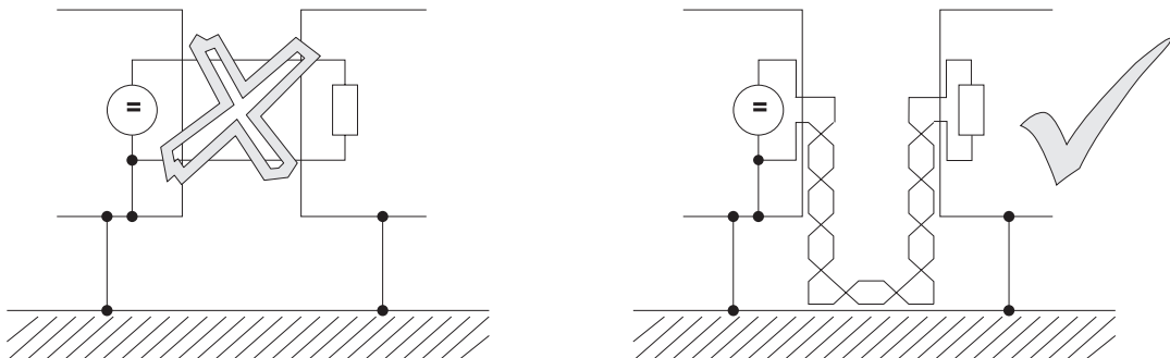
Abbildung 4: Leitungsverlegung - Schleifenfläche
