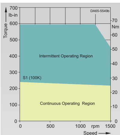
1FT6102-8AB7-....
