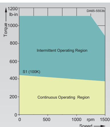
1FT6105-8AB7-....
