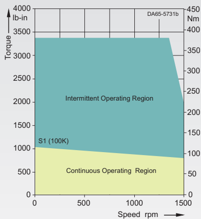
1FT6136-6AB7-....
