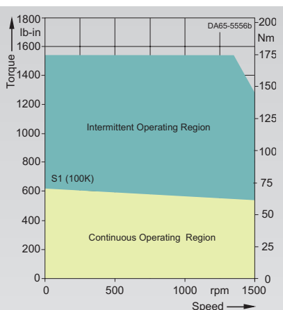
1FT6108-8AB7-....
