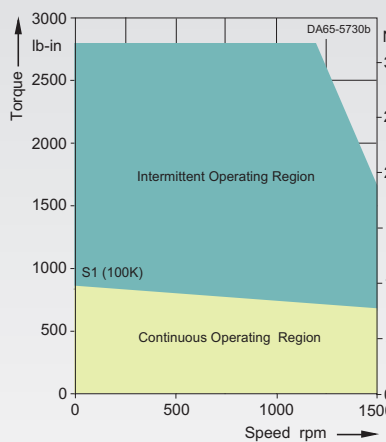
1FT6134-6AB7-....
