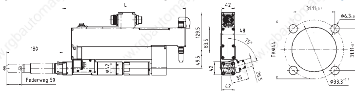
versetzter Abtrieb, 1 Messwertaufnehmer / Offset drive, single transducer
