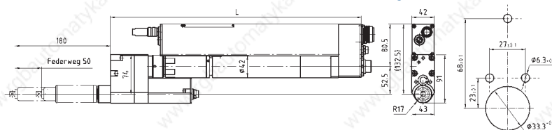
versetzter Abtrieb mit Motor-Umlenkgetriebe, 1 Messwertaufnehmer / Offset drive with reversible gears, single transducer
