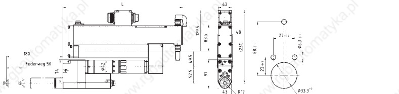
Winkelabtrieb, 1 Messwertaufnehmer / Angle drive, single transducer
