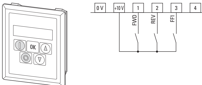
Ilustracja 69: Opcjonalny panel obsługi DXE-KEY-LED i zaciski sterowania P-15 = 0 (nastawa fabryczna, Mode 0)
