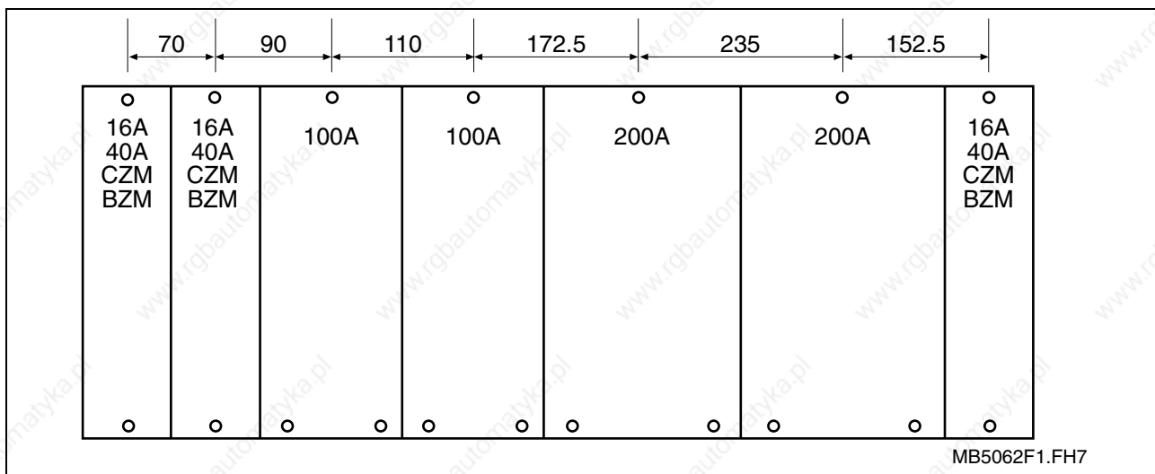
Fig. 12-16: Module widths
