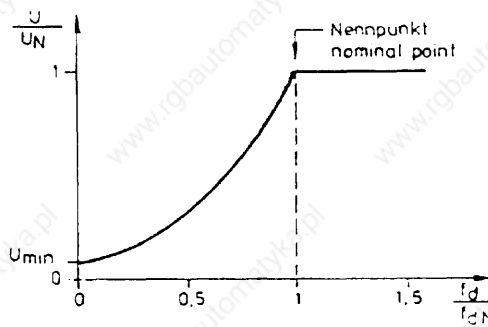
quadratische Kennlinie square characteristic
