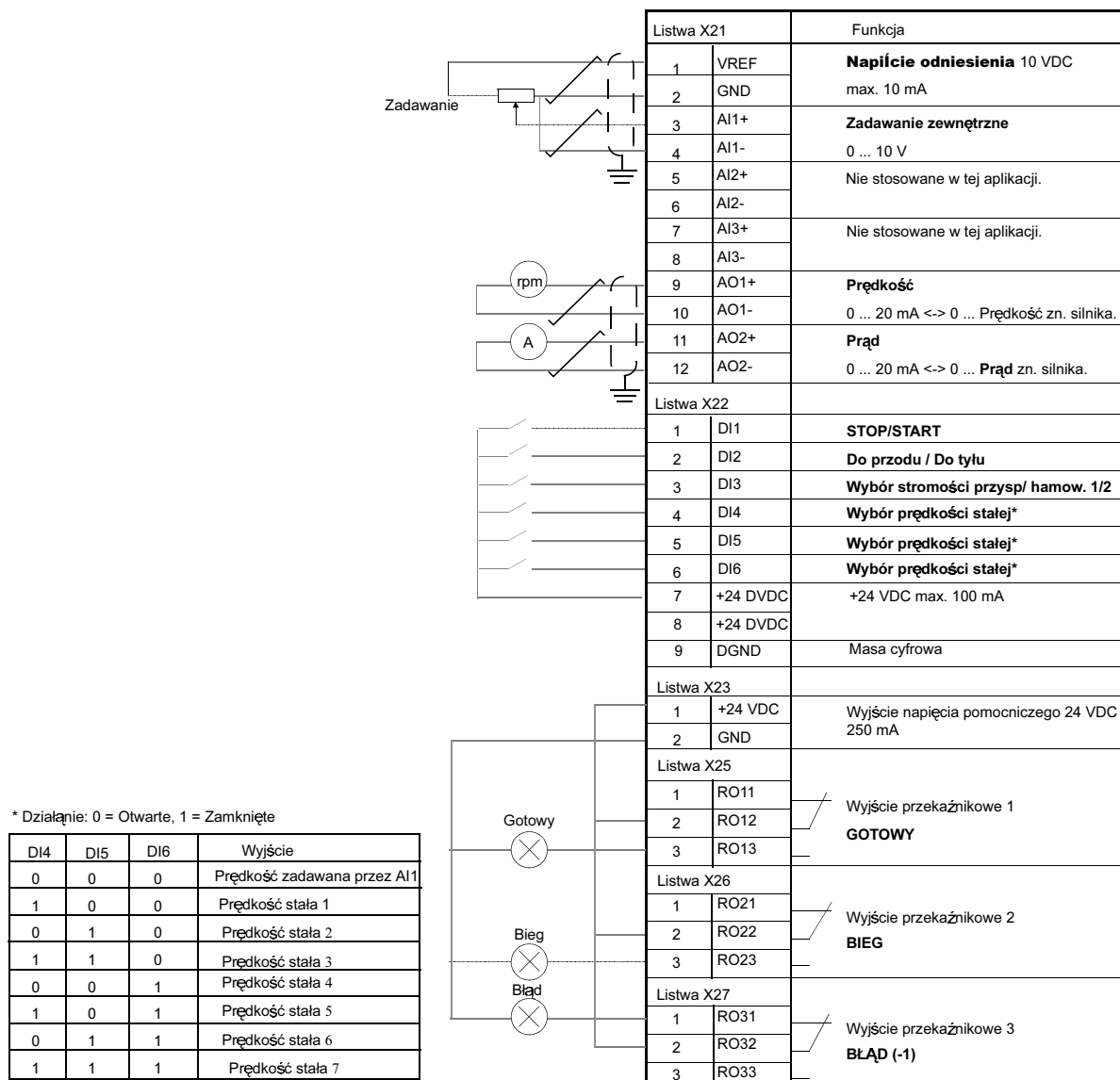
Rysunek 5-15 : Połączenia sterujące dla Makroaplikacji STEROWANIE SEKWENCYJNE . Oznaczenia złącz płyty NIOC przedstawiono powyżej. W ACS 601 i ACS 604 połączenia użytkownika są zawsze wykonane bezpośrednio do zacisków wejścia i wyjścia płyty NIOC. W ACS 607 połączenia te są wykonywane albo bezpośrednio do płyty NIOC albo zaciski We/Wy płyty NIOC są wyprowadzone na oddzielną listwę przeznaczoną na połączenia użytkownika - właściwe oznaczenia zacisków patrz odpowiedni podręcznik instalacji i uruchamiania.
