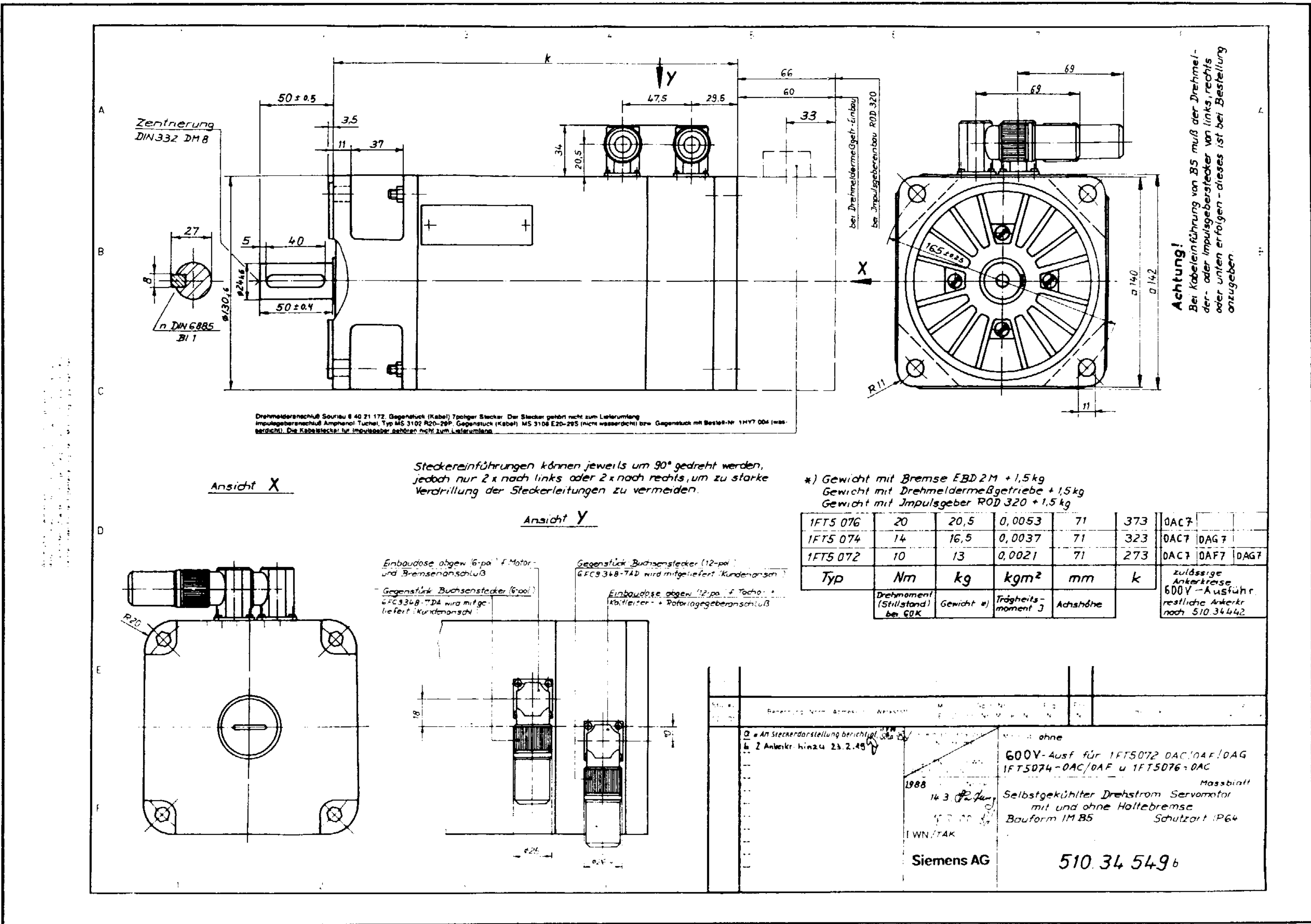
Bild 6.44 Maßblatt Drehstrom-Servomotoren 1FT5072-0AC/0AF/0AG, 1FT5074-0AC/0AF und 1FT5076-0AC mit Option Steckerausführung
