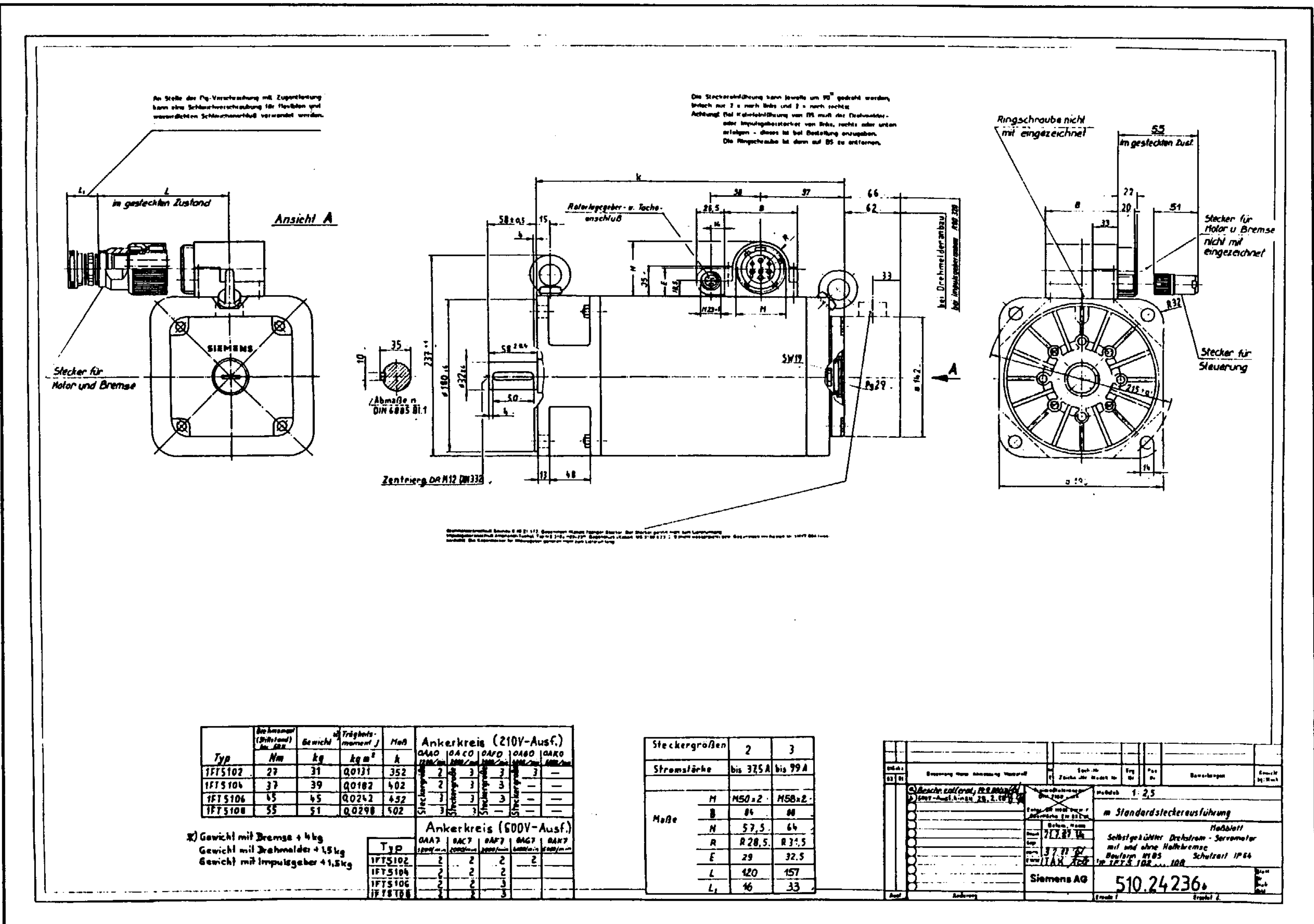
Bild 6.45 Maßblatt Drehstrom-Servomotoren 1FTS102 bis 1FTS108 mit Option Steckeranführung IM B5 Bitte achten Sie auf die Zuordnung der Klemmenkastengrößen für die Ankerkreise 600V. Bauform.
