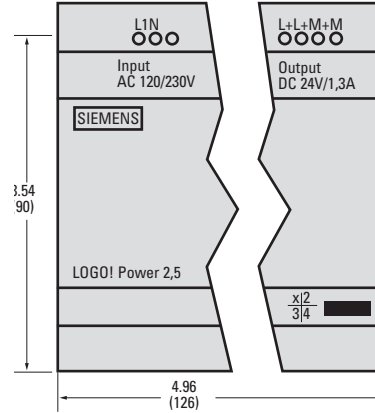
6EP1332-1SH41, DC 24V/2.5A
