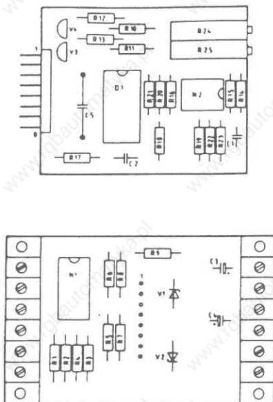
Bestückungsplan
