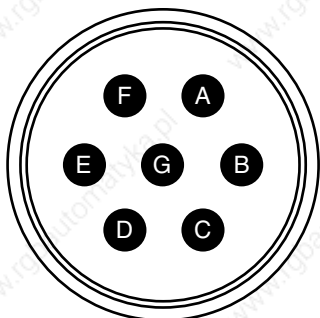
FRAME 142 & 190 – MS3102E-24-10P
