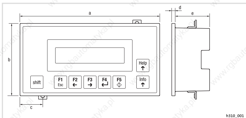
Fig.2-2 Encombremments
