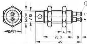
Type RFL-4
