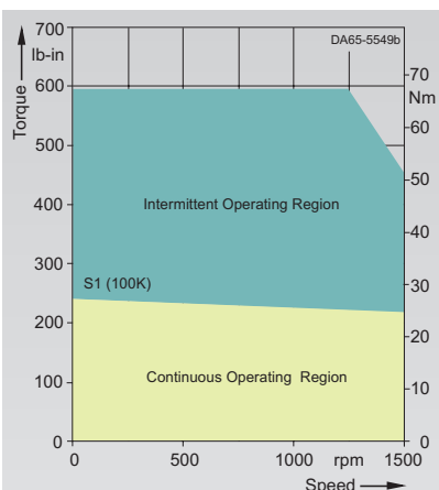
1FT6102-8AB7-....
