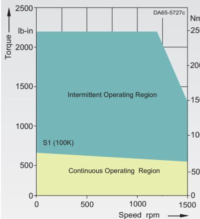
1FT6132-6AB7-....
