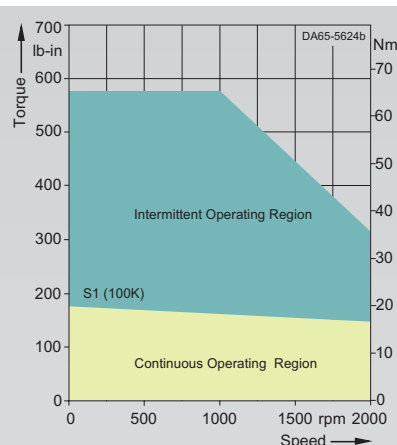
1FT6084-8AC7-....
