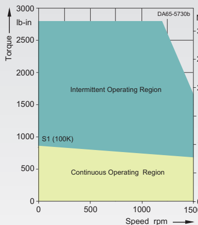
1FT6134-6AB7-....
