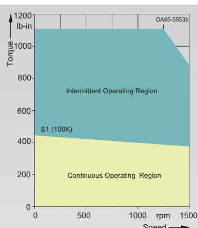
1FT6105-8AB7-....
