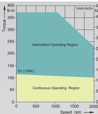
1FT6082-8AC7-....
