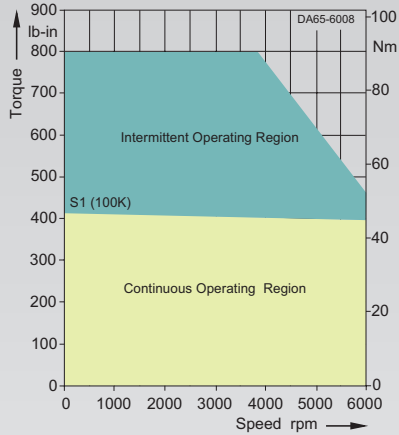
1FT6086-8WK7-.....
