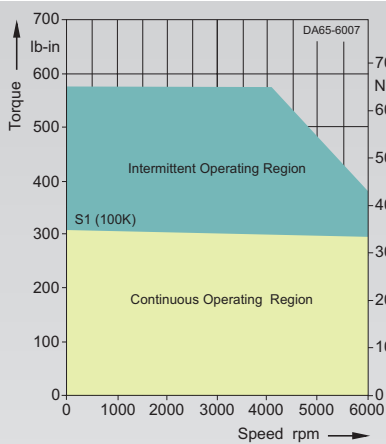
1FT6084-8WK7-.....
