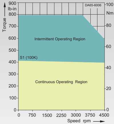
1FT6086-8WH7-.....
