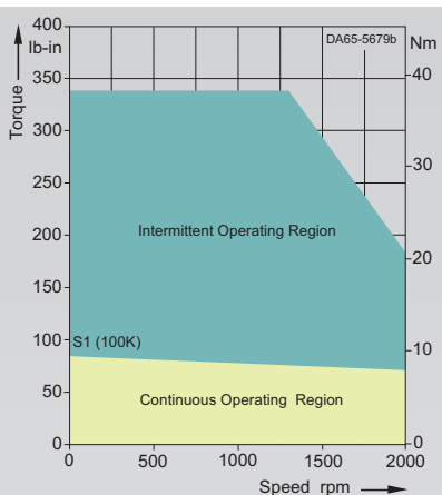
1FT6064-6AC7-....
