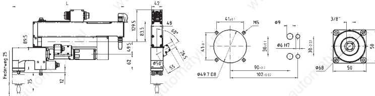
Winkelabtrieb mit Motor-Umlenkgetriebe, 2 Messwertaufnehmer / Angle drive with reversible gears, twin transducer (redundant)
