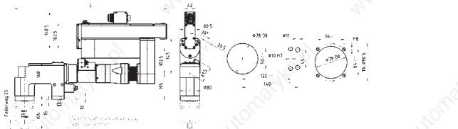
Winkelabtrieb mit Motor-Umlenkgetriebe, 2 Messwertaufnehmer / Angle drive with reversible gears, twin transducer (redundant)
