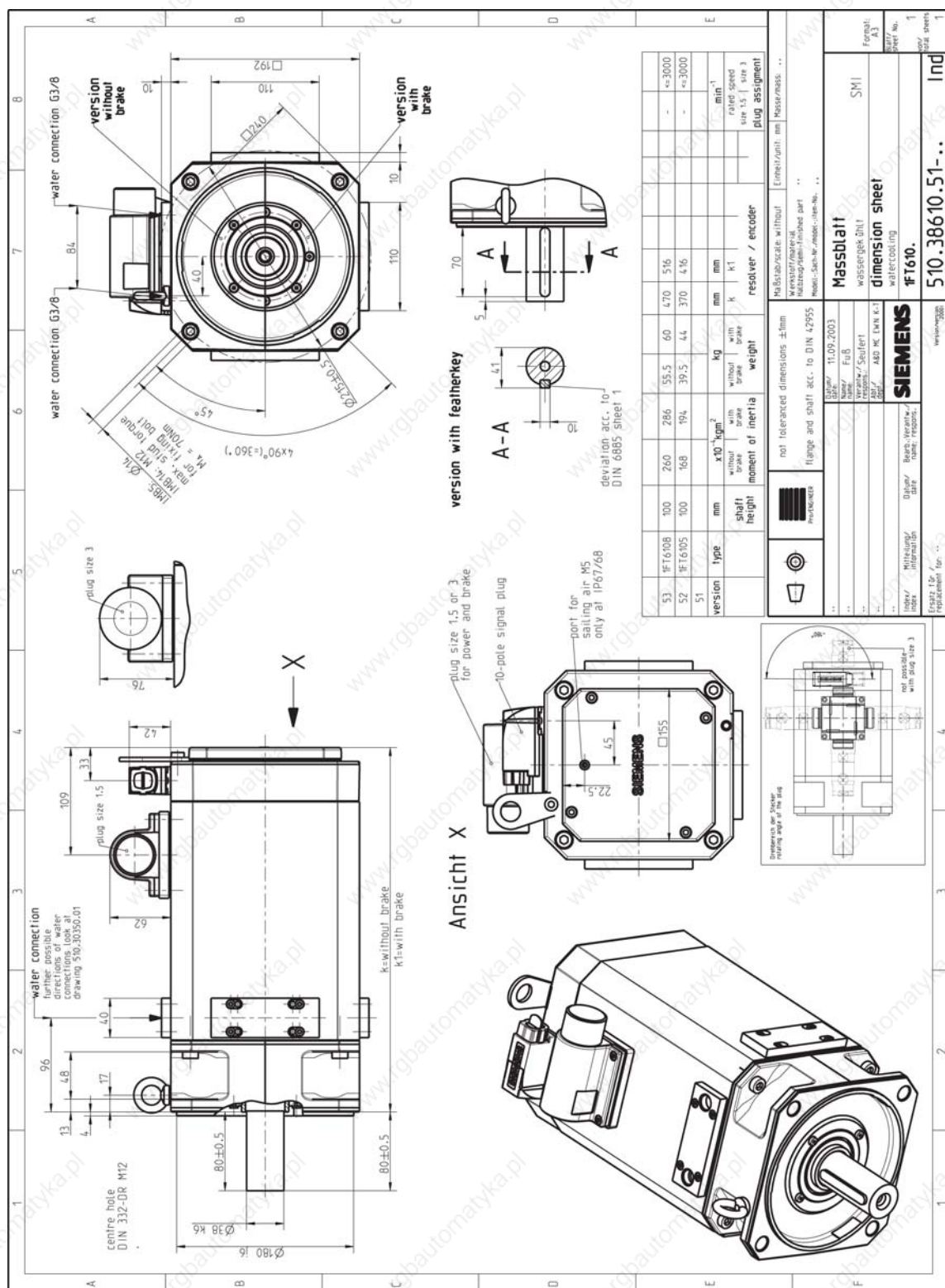
Figure 5-14 1FT610□-□W□plug□DQ
